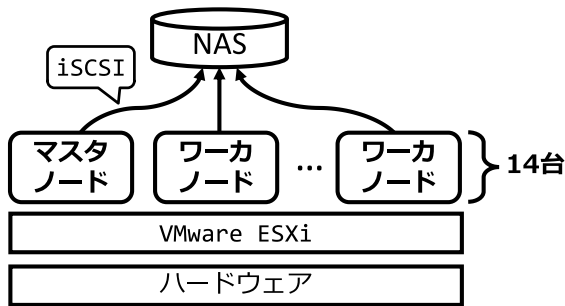
図 10 システムアーキテクチャ
