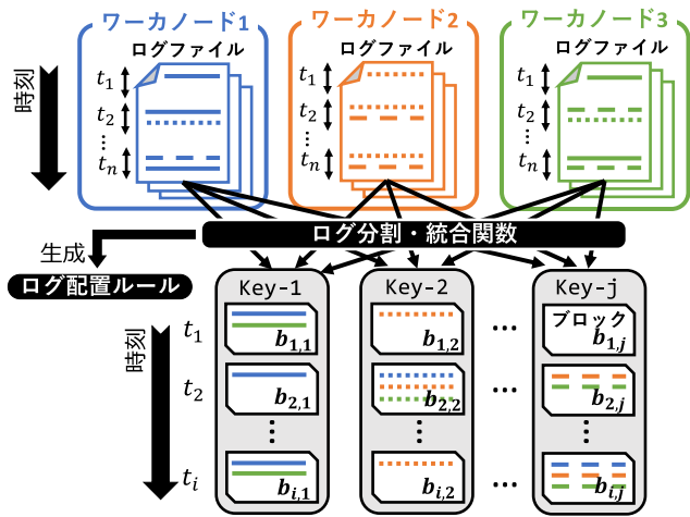
図 6 ブロックの作成
